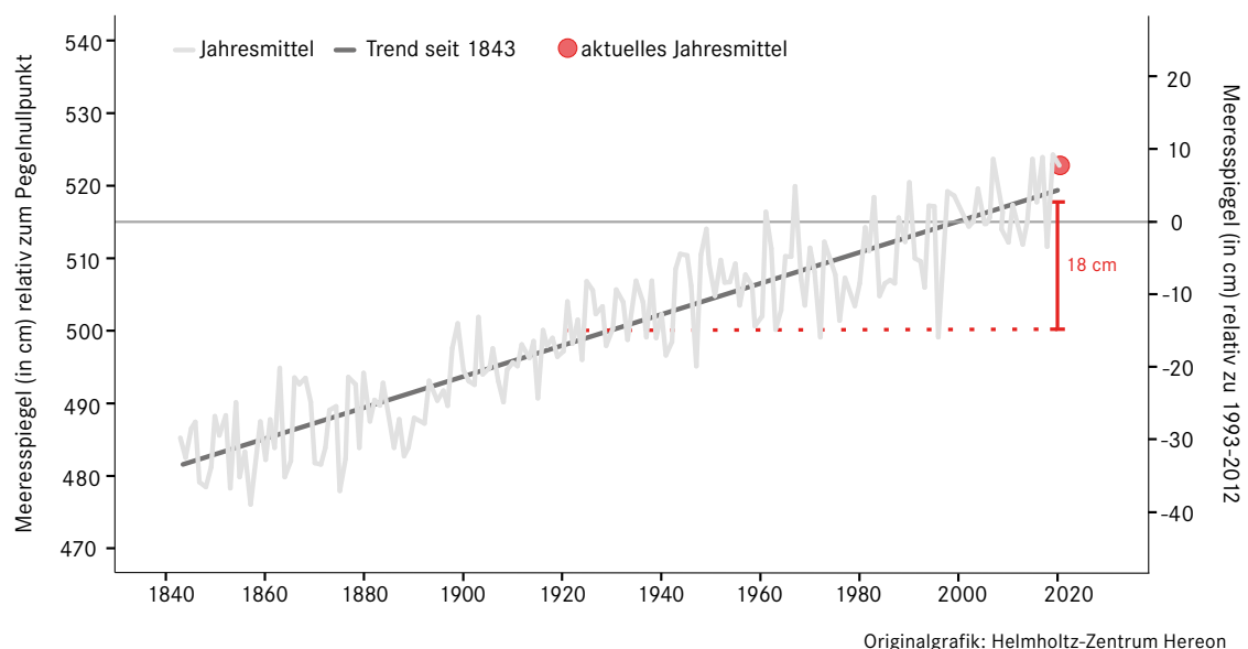
MEERESSPIEGELANSTIEG SEIT 1843 PEGEL CUXHAVEN
