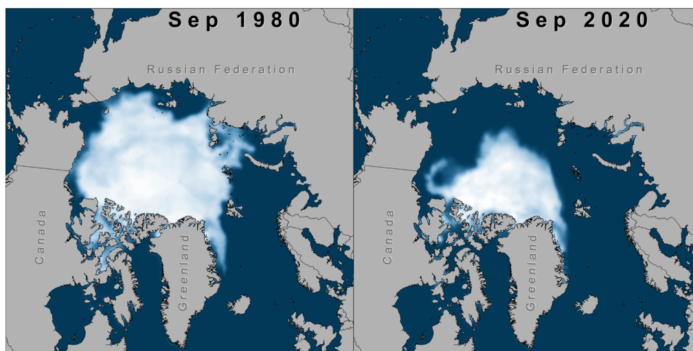
MEEREISFLÄCHE IM POLARMEER
